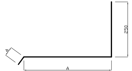
NO13 : EDGE STRIP
