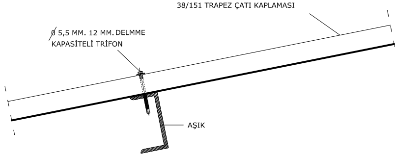
AŞIĞA MONTAJ DETAYI
