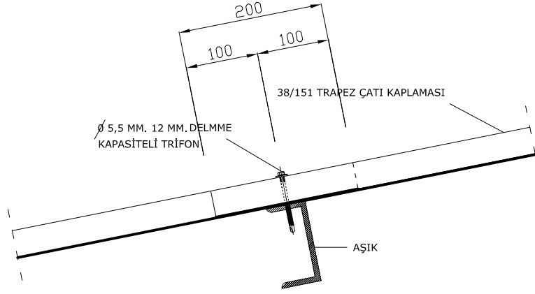
EK YERİ MONTAJ DETAYI
