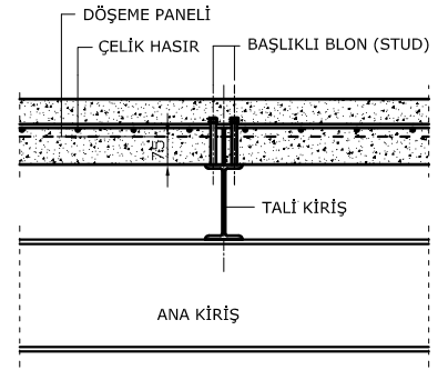
C-C KESİTİ (DÖŞEME PANELİ EK YERİ DETAYI)
