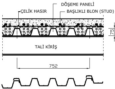
A-A KESİTİ
