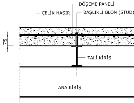
B-B KESİTİ
