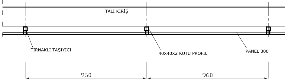
B-B KESİTİ
