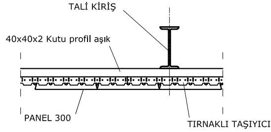
A-A KESİTİ
